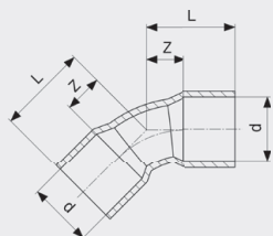
Отвод 45° - медь Модель 95041
