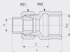
Соединительный элемент резьбовой разъемный Модель 94340G
