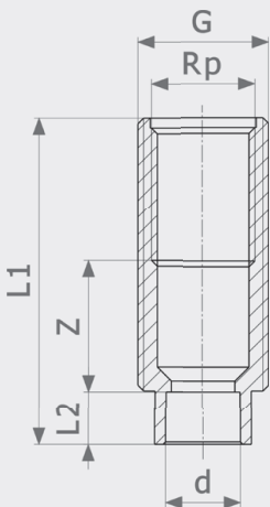
Водорозетка - бронза Модель 3427.2
