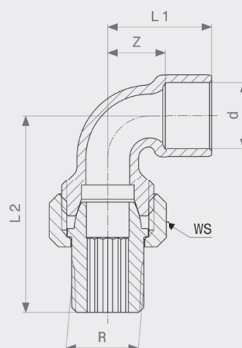
Переходной элемент 90° Модель 94098G
