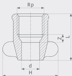
Соединительный элемент - бронза Модель 94270GF
