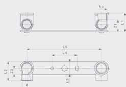
Монтажный узел Gemini Модель 94476.05
