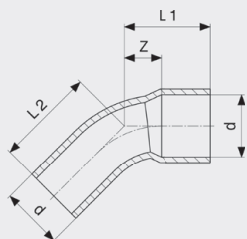
Отвод 45° - медь Модель 95040
