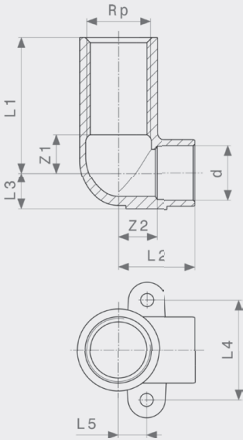
Водорозетка - бронза Модель 94472GL
