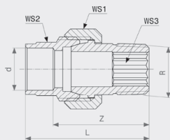
Соединительный элемент резьбовой разъемный Модель 94341G
