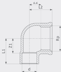
Угольник переходной 90° - бронза Модель 94090G
