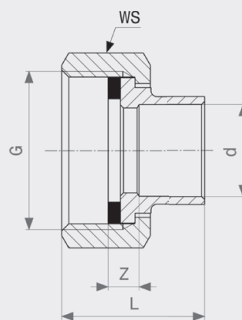
Переход на резьбовые соединения Модель 94359
