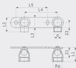
Монтажный узел Gemini Модель 94476.21
