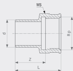
Соединительный элемент - бронза Модель 94246G
