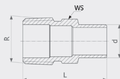
Соединительный элемент - бронза Модель 94280G
