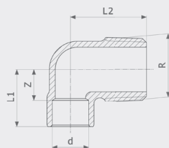
Угольник переходной 90° - бронза Модель 94092G
