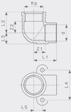
Водорозетка - бронза Модель 94472G
