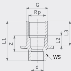
Водорозетка - бронза Модель 3427.1
