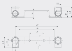
Монтажный узел Gemini Модель 94476.0
