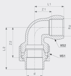
Переходной элемент 90° Модель 94096G
