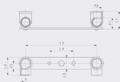
Монтажный узел Gemini Модель 94476.05NOR
