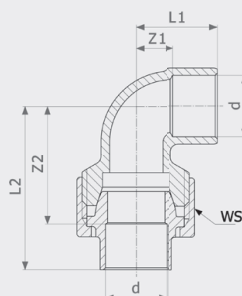
Переходной элемент 90° - бронза Модель 94096
