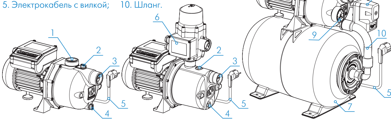
Поверхностный насос
