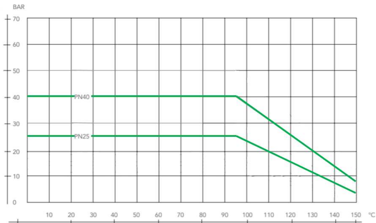
График зависимости температуры от рабочего давления
