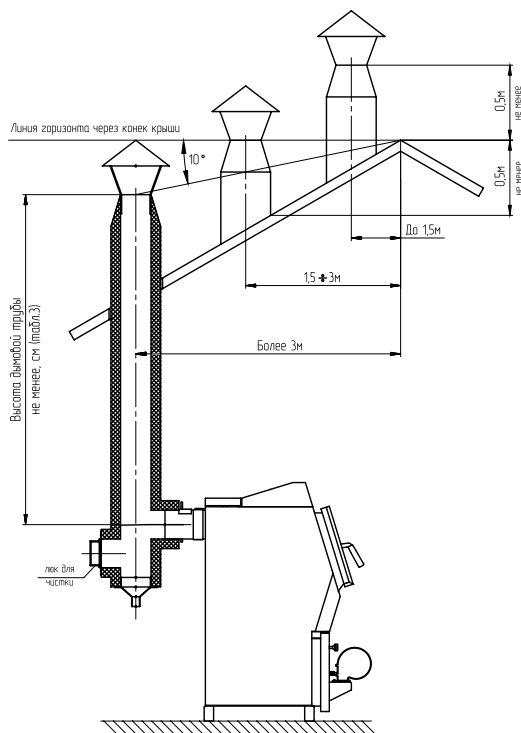
Рис.5 Варианты установки дымовой трубы
