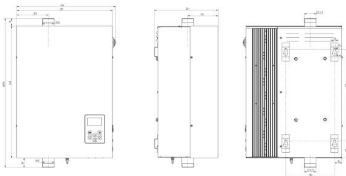
Габаритные и присоединительные размеры 30П-45П
