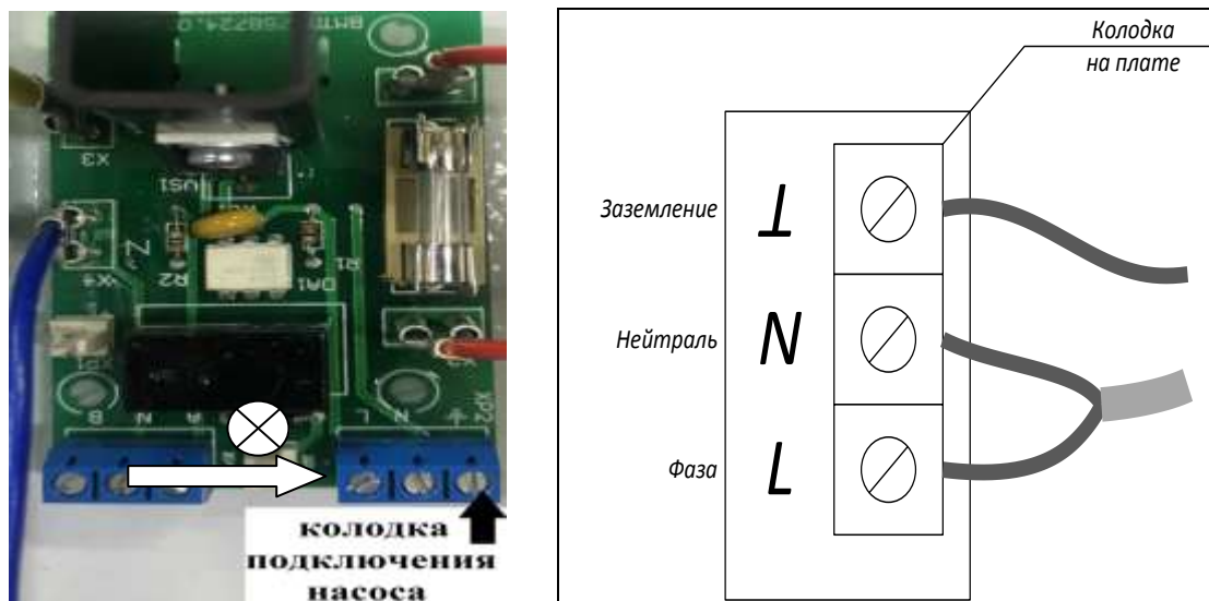
Рисунок 7. Подключение циркуляционного насоса к отопителю
