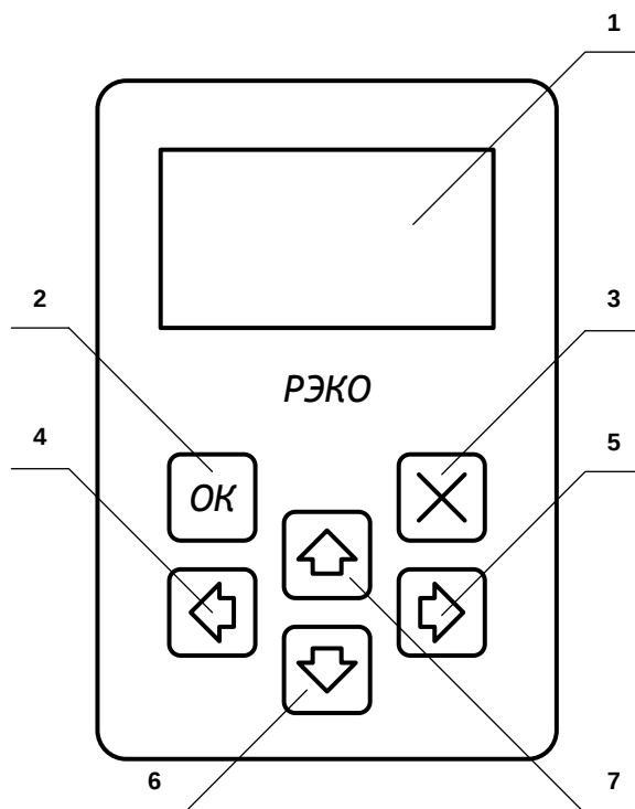
Рисунок 12. Внешний вид панели управления отопителя
