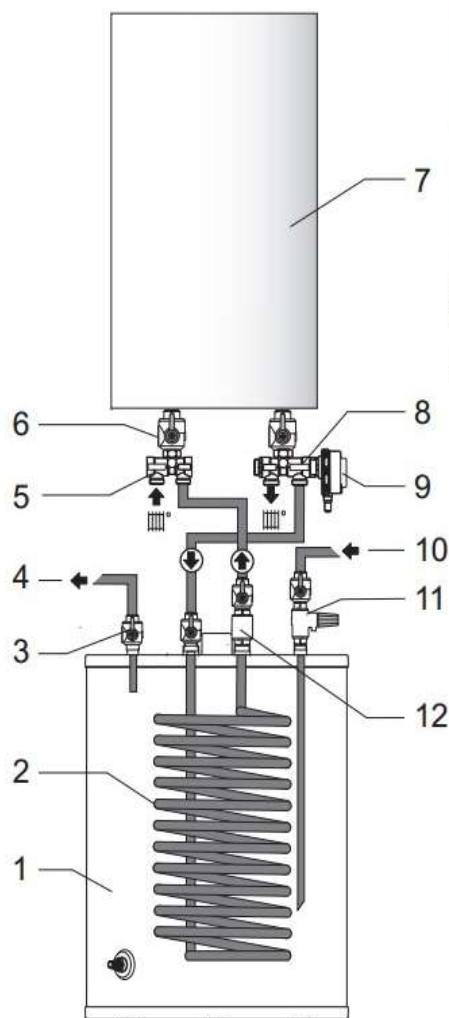
Рисунок 15. Типовая схема подключения бойлера косвенного нагрева
