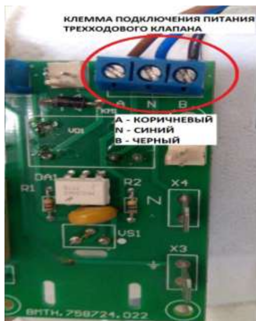
Рисунок 13. (плата управления насоса)
