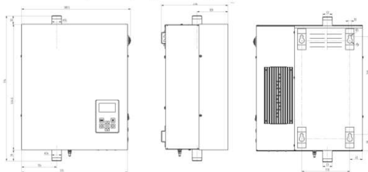
Габаритные и присоединительные размеры 12П-24П
